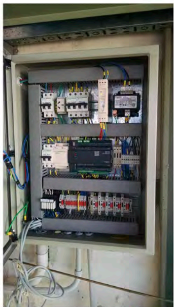
Armado de tablero electrico con PLC
